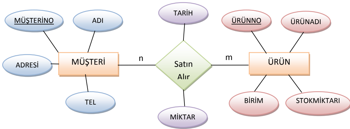
Şekil X: Müşteri-Ürün Satın alır n-m ilişkisi
